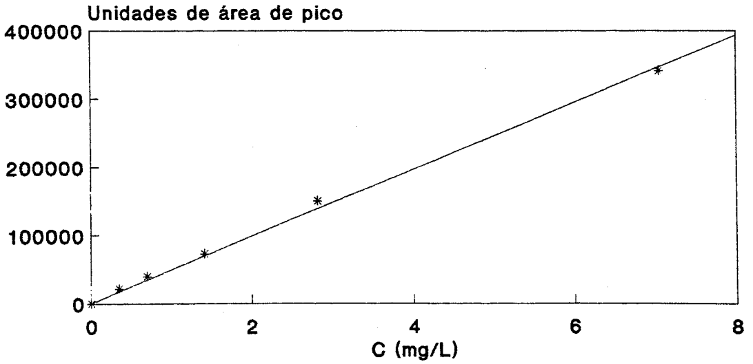
Figura 5 Valores de área de pico en función de la concentración de procimidona
