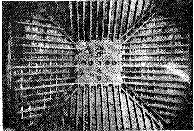
2. Armadura de lima cuadrada. Presbiterio de la iglesia parroquial de Instinción.
