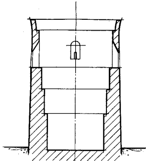
sección
