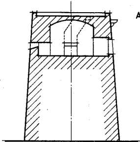
sección
