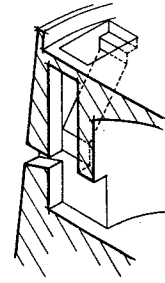
detalle de acceso a cubierta
