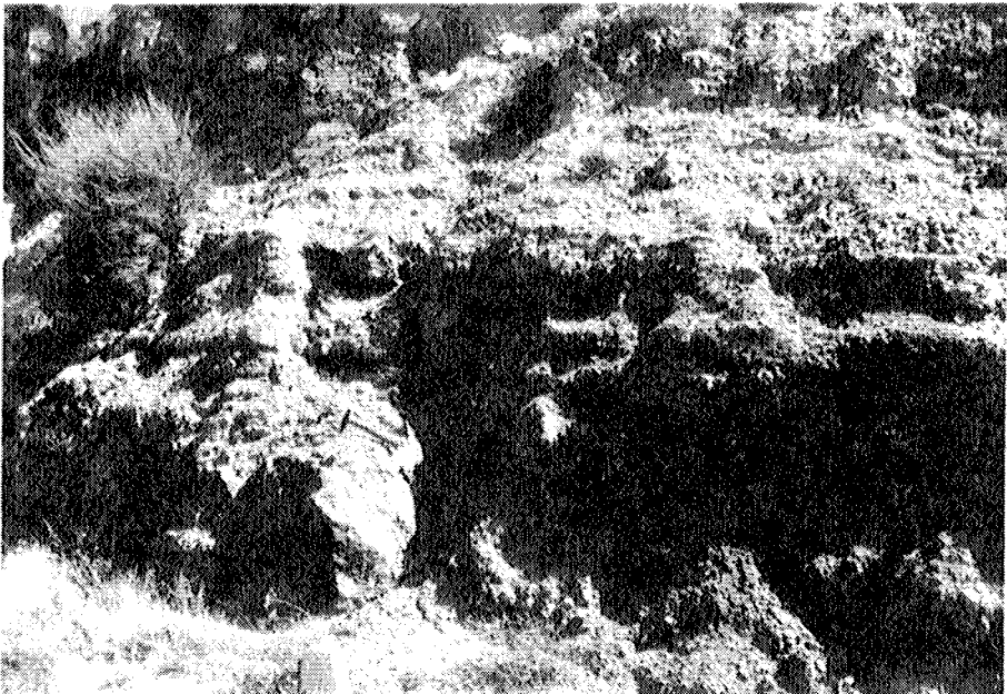
Fig. 11.— Aspecto del conglomerado basal (depósitos de abanico aluvial) tal como están expuestos en la Ctra. local de Vicar a Felix. Se aprecia la alternancia de lechos de conglomerados y lutitas. El martillo señala un gran bloque dolomítico ( \pm 1 metro de eje mayor). (Foto L. Delgado.)
