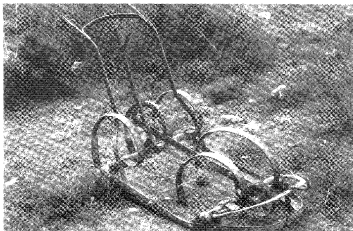
Arado calariense de cinco rejas
