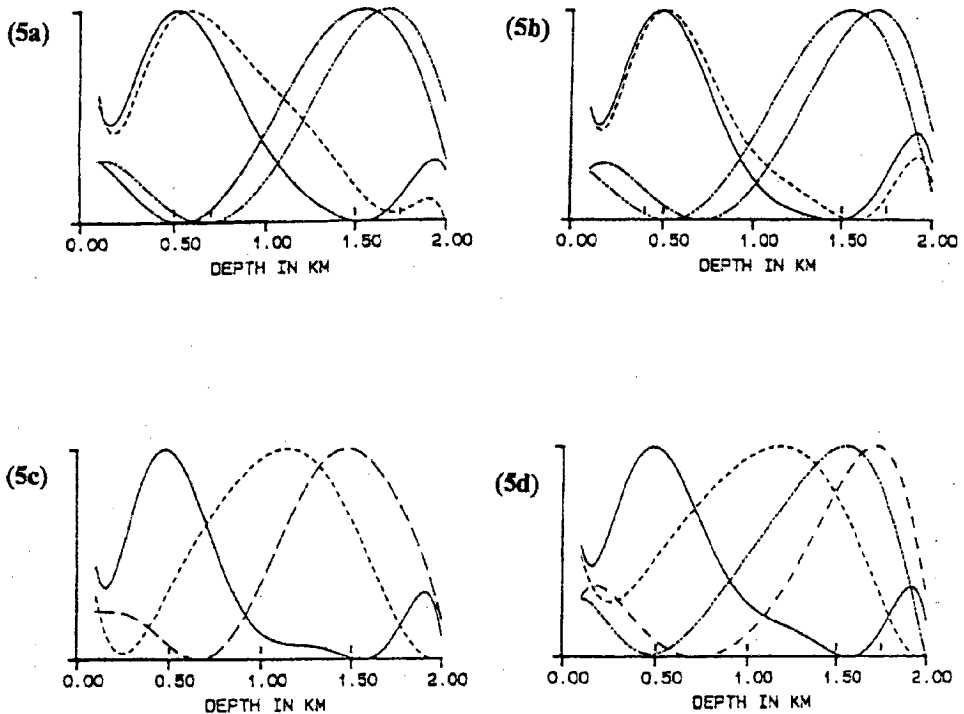
FIG. 5.- Núcleos de resolución del modelo de velocidad compresional para diferentes profundidades de referencia.
