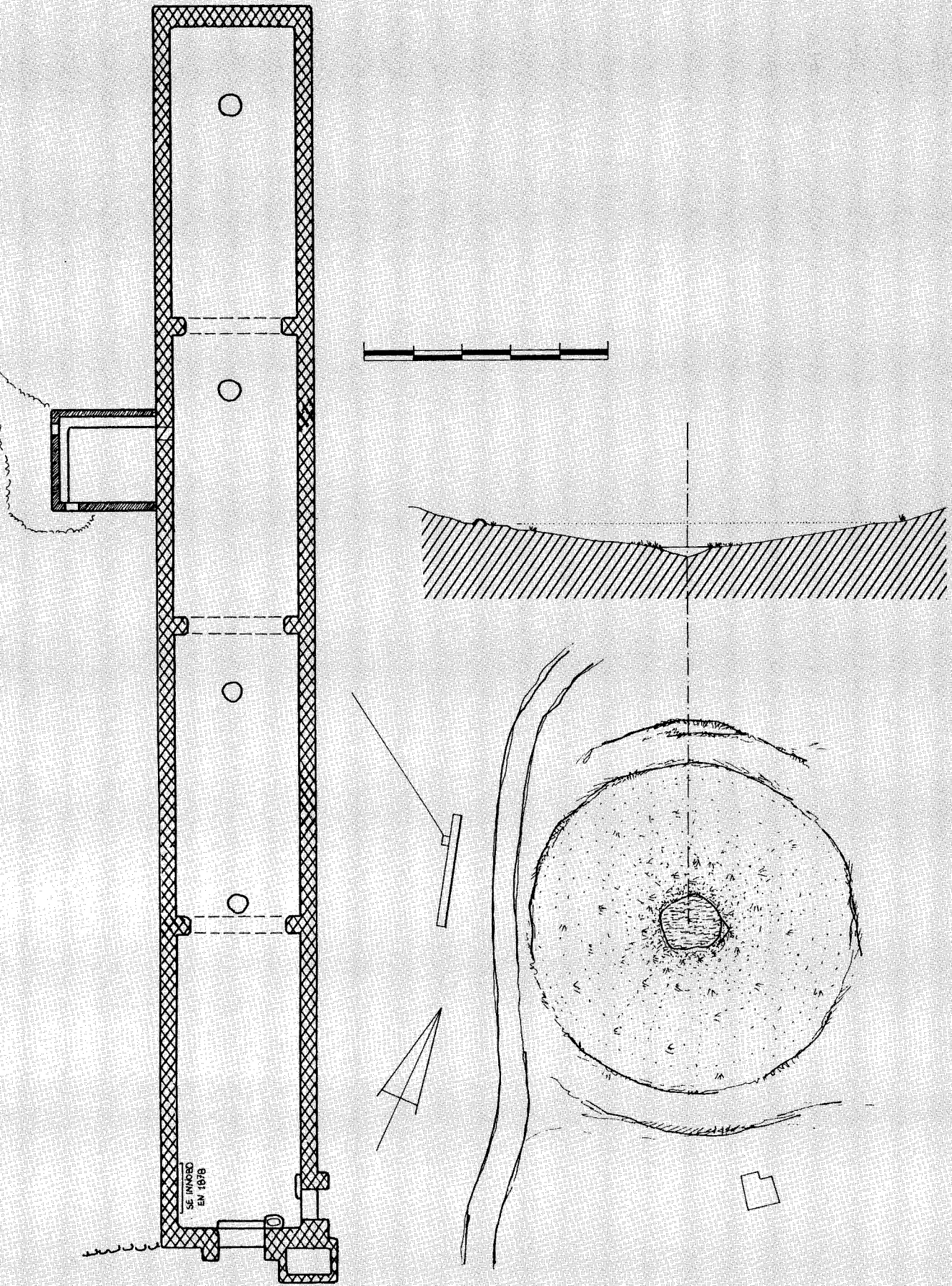
Planta del ajiibe de La Chanata y balsón inmediato.
