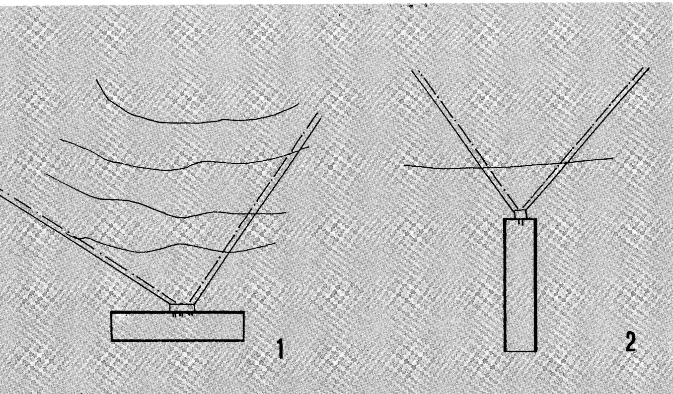
Fig. 1. Aljibe de relieve. La admisión de agua es rápida y violenta. Tienen que situar la entrada transversal formada por varios agujeros pequeños, que impidan la entrada de material grueso, por eso se sitúa en el lado más sólido.
