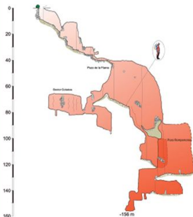
PERFIL
